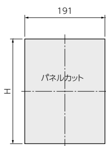
パネルカット寸法 (単独取付)
