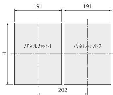
(パネルカット1と2のセンターピッチ)
