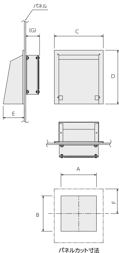
パネルカット寸法
