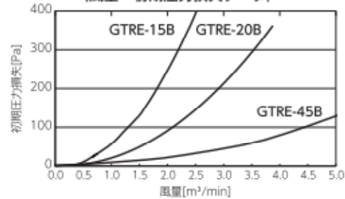
〈風量—初期圧力損失データ〉
