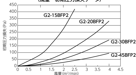
〈風量－初期圧力損失データ〉
