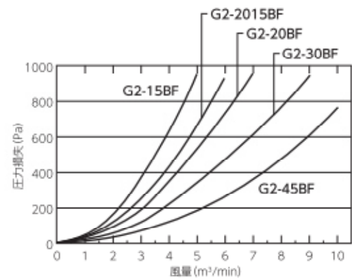
〈風量—初期圧力損失データ〉
