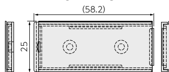
カバー部“閉”状態寸法
