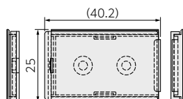
カバー部“閉”状態寸法
