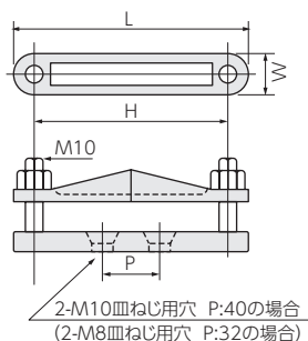
水平クランプC2H型（2本止）
