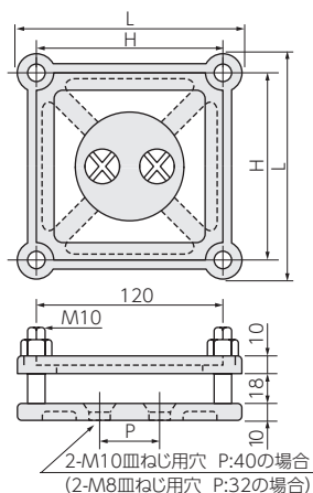
水平クランプC4H型（4本止）
