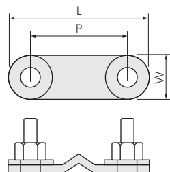
丸線クランプCB型（丸穴）
