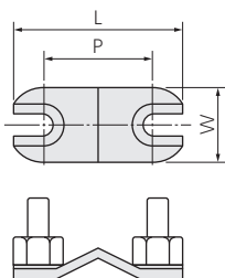
丸線クランプCA型（両切）
