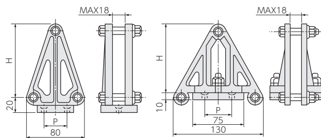
A型クランプCAE型（簡易型）
