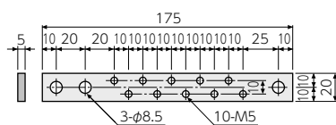
EBA-25-18タイプ
