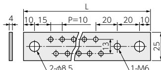
EBA-25タイプ
