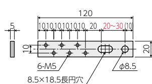
EBA-20-6タイプ
