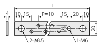
EBA-20タイプ
