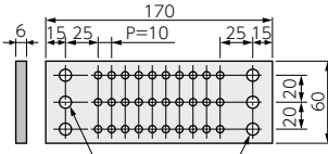
EBA-60タイプ
