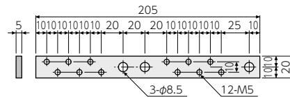
EBA-25-20タイプ
