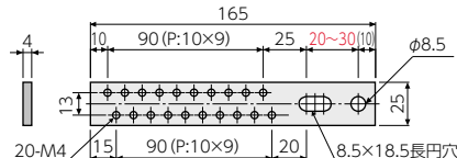
EBA-25-20タイプ
