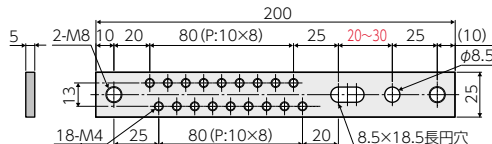
EBA-25-18タイプ
