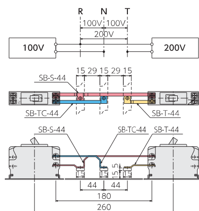
〔単相 100V、200V〕
