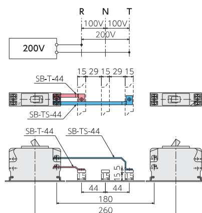
〔単相 200V〕
