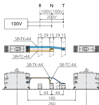
〔単相 100V〕
