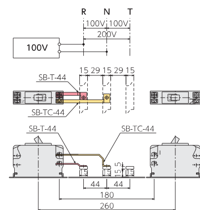
〔単相 100V〕
