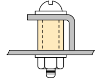
〈アングル補強例〉
