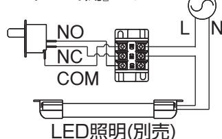
【使用例 (NC接点)】 ドア『開』でON
