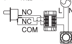
【使用例 (NO接点)】 ドア『閉』でON
