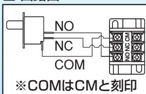
■ 回路図
