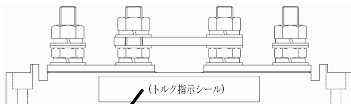
図 1：製品側面図
