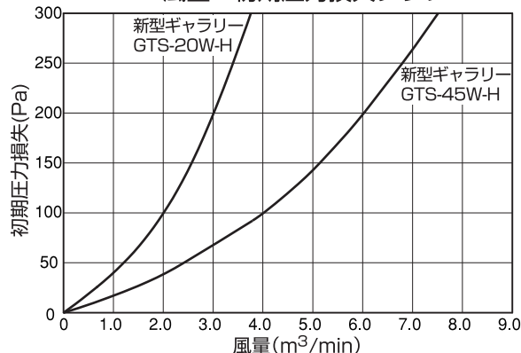
風量—初期圧力損失グラフ
