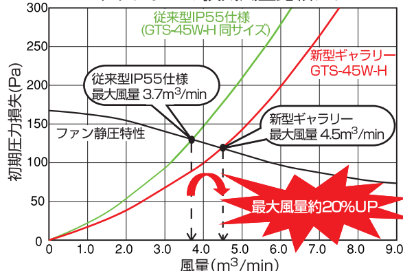
ギャラリの換気風量比較グラフ
