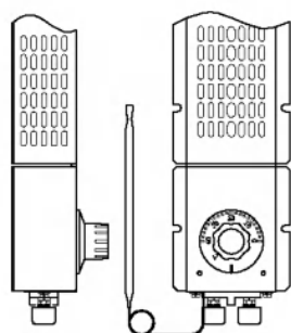
変更前 (2部品の締結構造)
