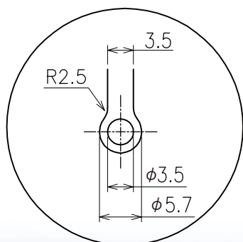
端子部形状
