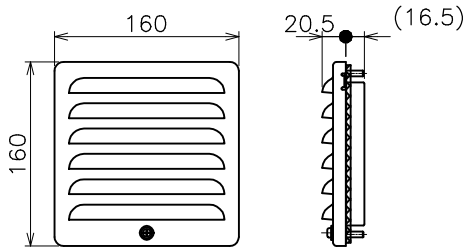
＜外形寸法図＞
