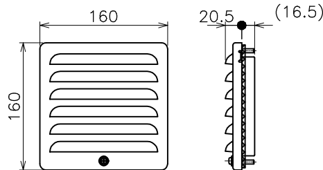
<外形寸法図>
