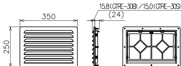
＜外形寸法図＞
