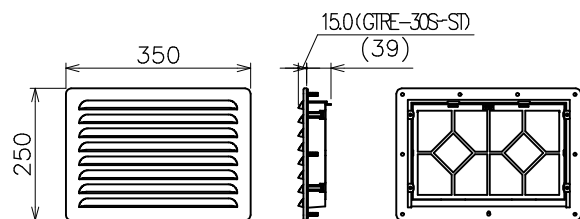
＜外形寸法図＞
