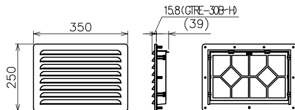
＜外形寸法図＞
